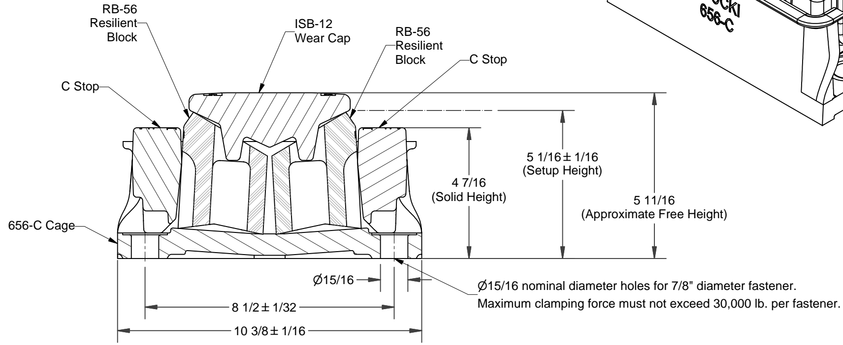
SECTION A-A
