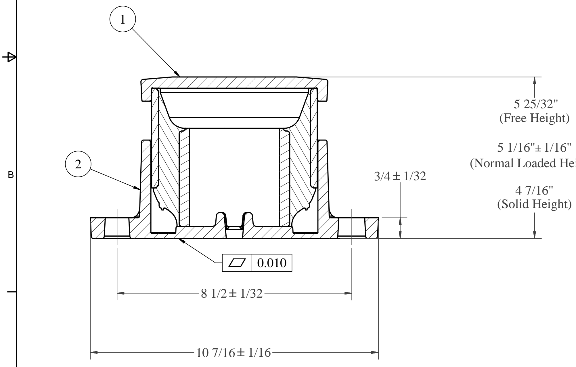
SECTION A-A
